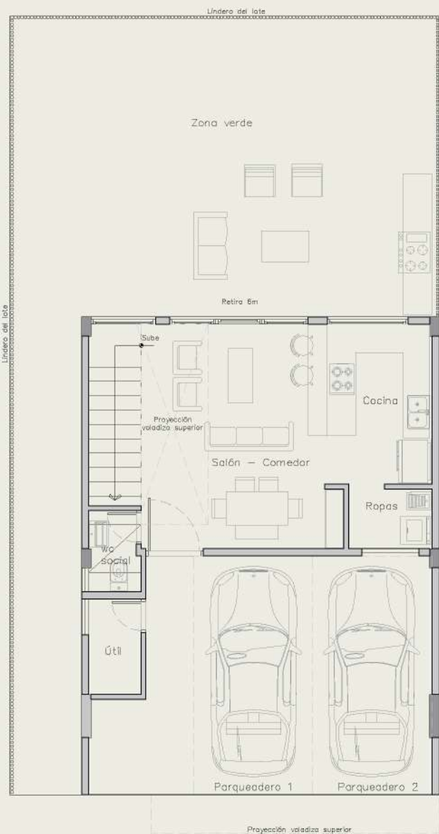
Planta primer piso Área 75m 2
