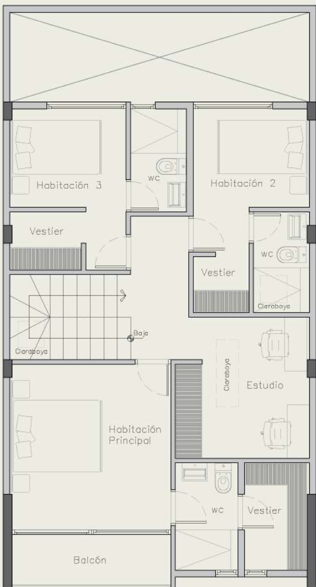
Planta segundo piso Área 70,55m 2 / Total 146,5 m 2
